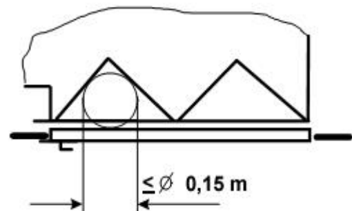
图5 铰链层门和折叠轿门的间隙
