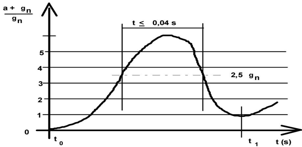
to—撞击缓冲器瞬间 (第1个绝对值最小时); t1—第2个绝对值最小时 图F1 减速图
