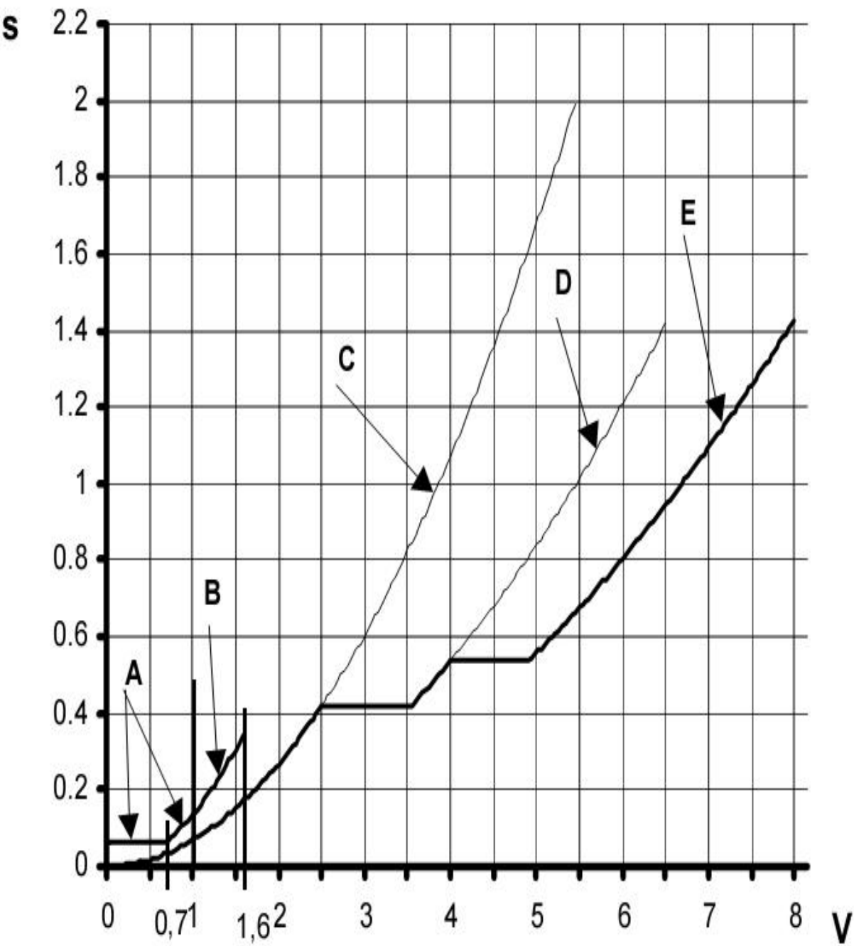
S —缓冲行程, m; v —( )—额定速度, m/s; ①—蓄能型缓冲器(10.4.1.1); ②—(略); ③—无减行程的耗能型缓冲器(10.4.3.1); ④—减至50%行程的耗能型缓冲器[10.4.3.2a]; ⑤—减至1/3行程的耗能型缓冲器[10.4.3.2b]; ⑥—粗线表示采用10.4.3的所有可能性有利条件而得到的最小可能缓冲行程
