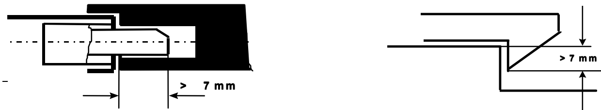
图3 锁紧元件示例
