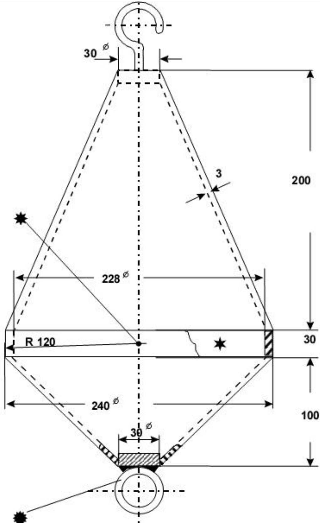
①—冲击环；②—测量跌落高度参考点；③—触发装置附件 图 J1 硬摆锤冲击装置
