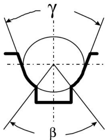
图 M1 带切口的圆槽
